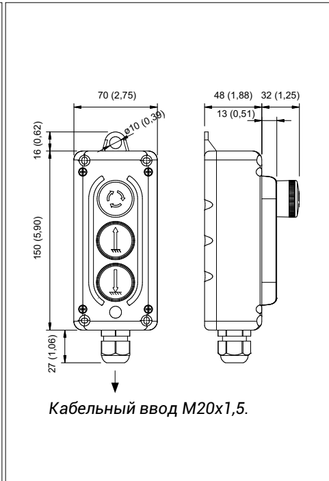
ТЕХНИЧЕСКИЙ ЧЕРТЕЖ – TLP3.B
