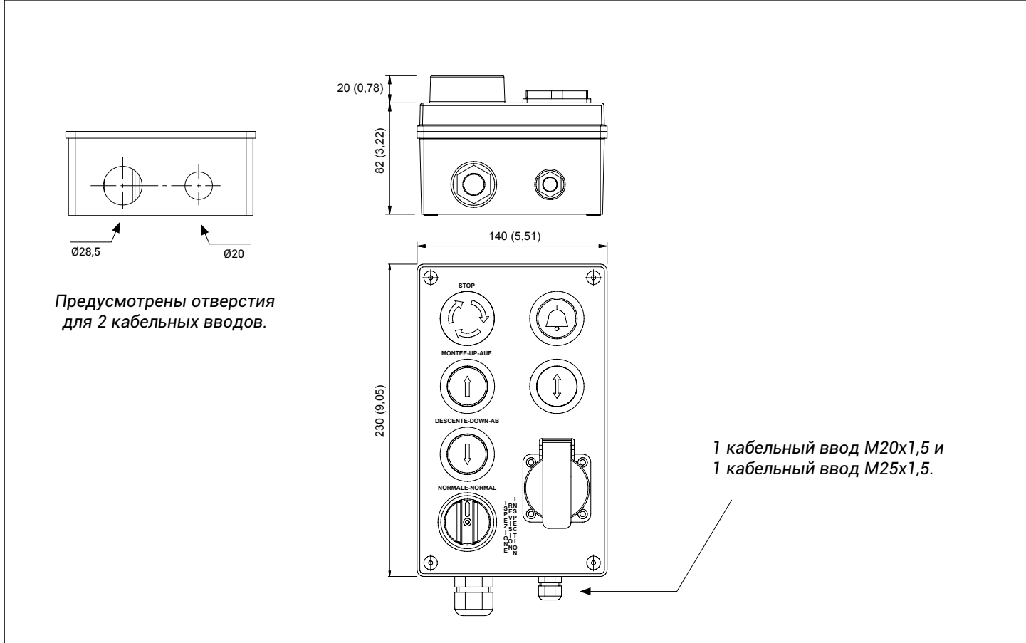
ТЕХНИЧЕСКИЙ ЧЕРТЕЖ – GM412BK/..
