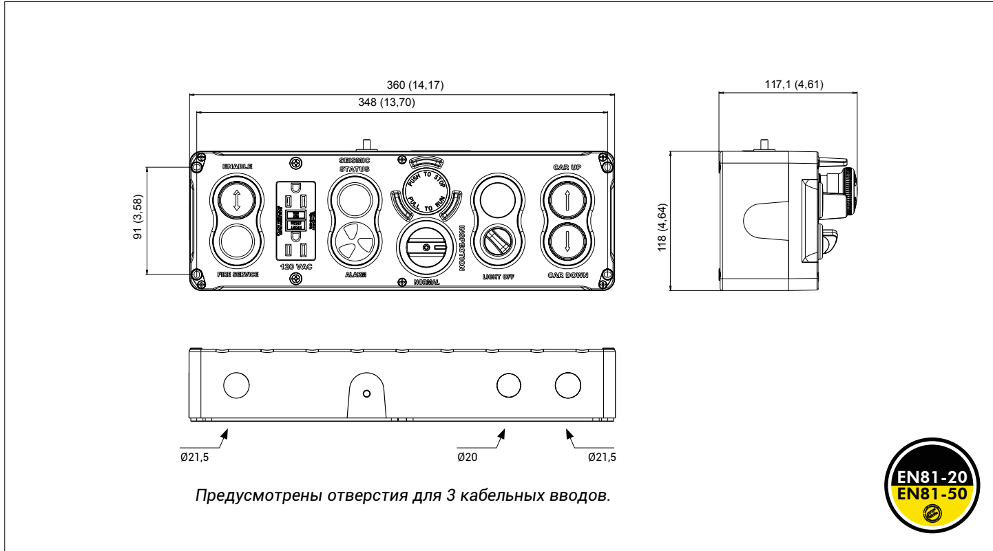
ТЕХНИЧЕСКИЙ ЧЕРТЕЖ – GMS305
