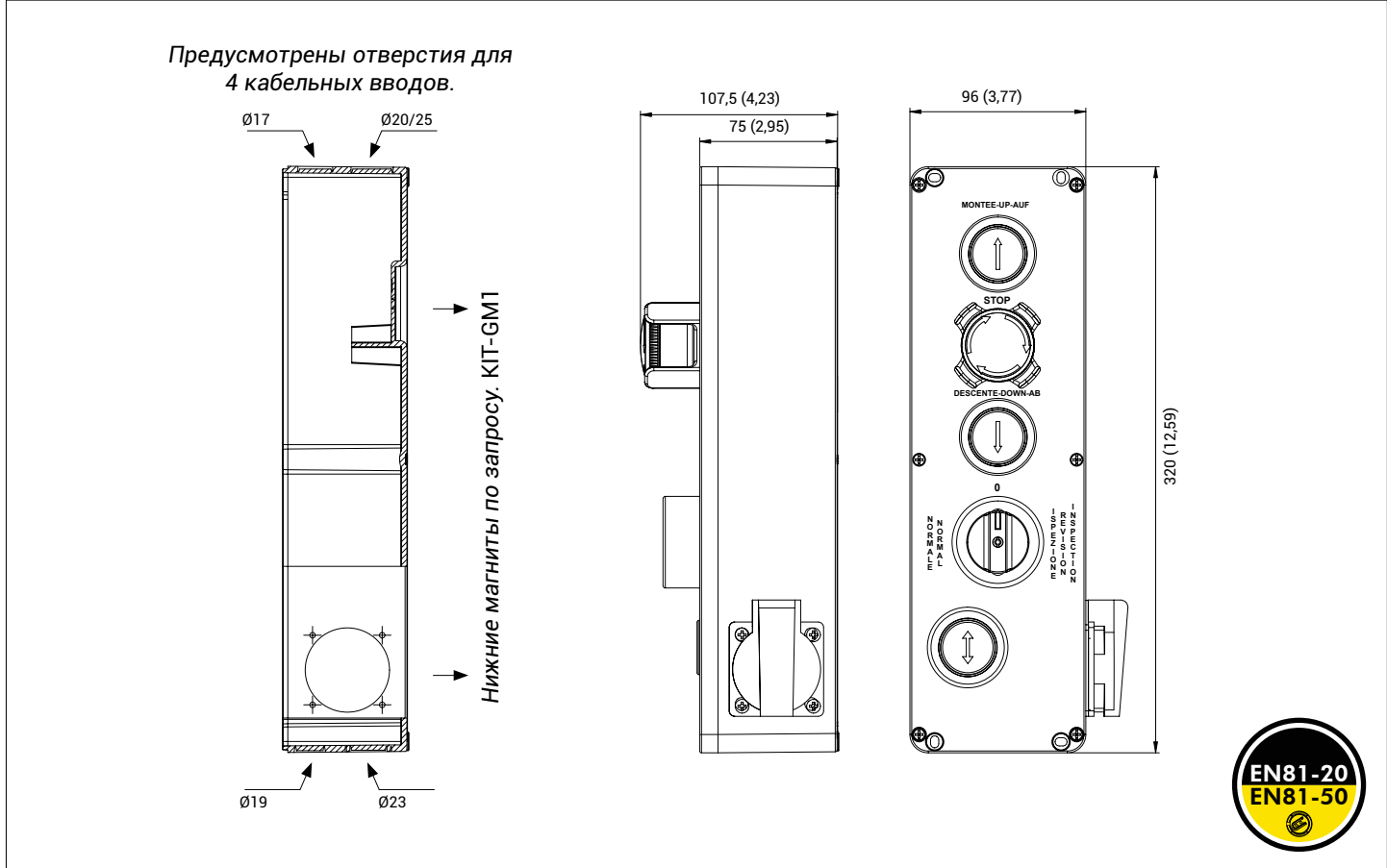
ТЕХНИЧЕСКИЙ ЧЕРТЕЖ – GM677/..
