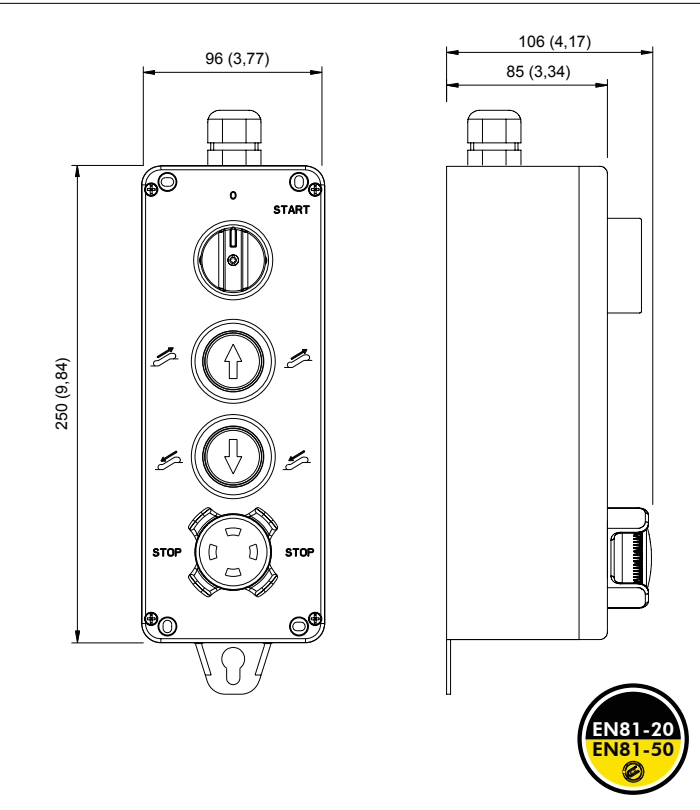
ТЕХНИЧЕСКИЙ ЧЕРТЕЖ – GM245
