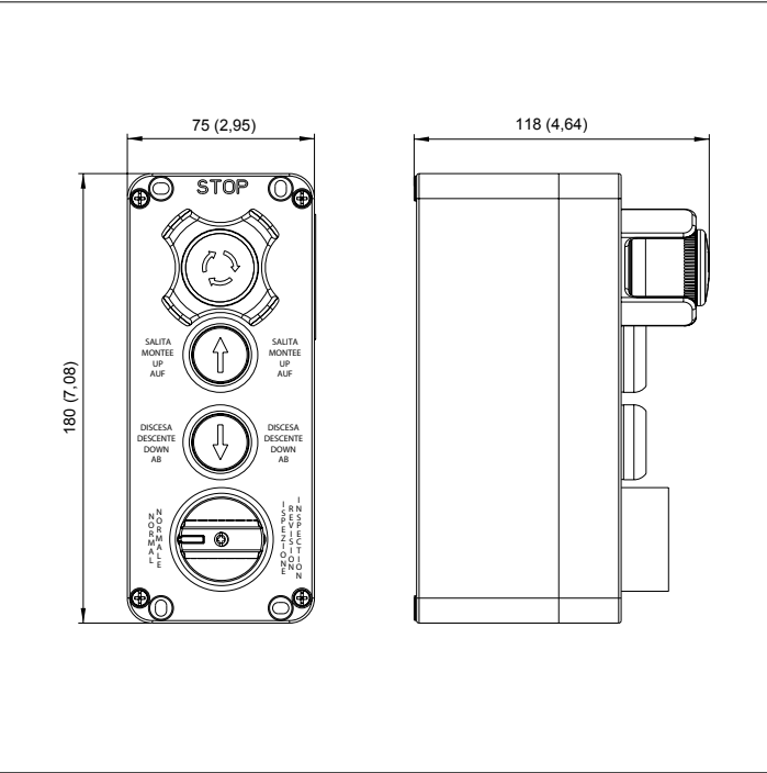
ТЕХНИЧЕСКИЙ ЧЕРТЕЖ – GM488
