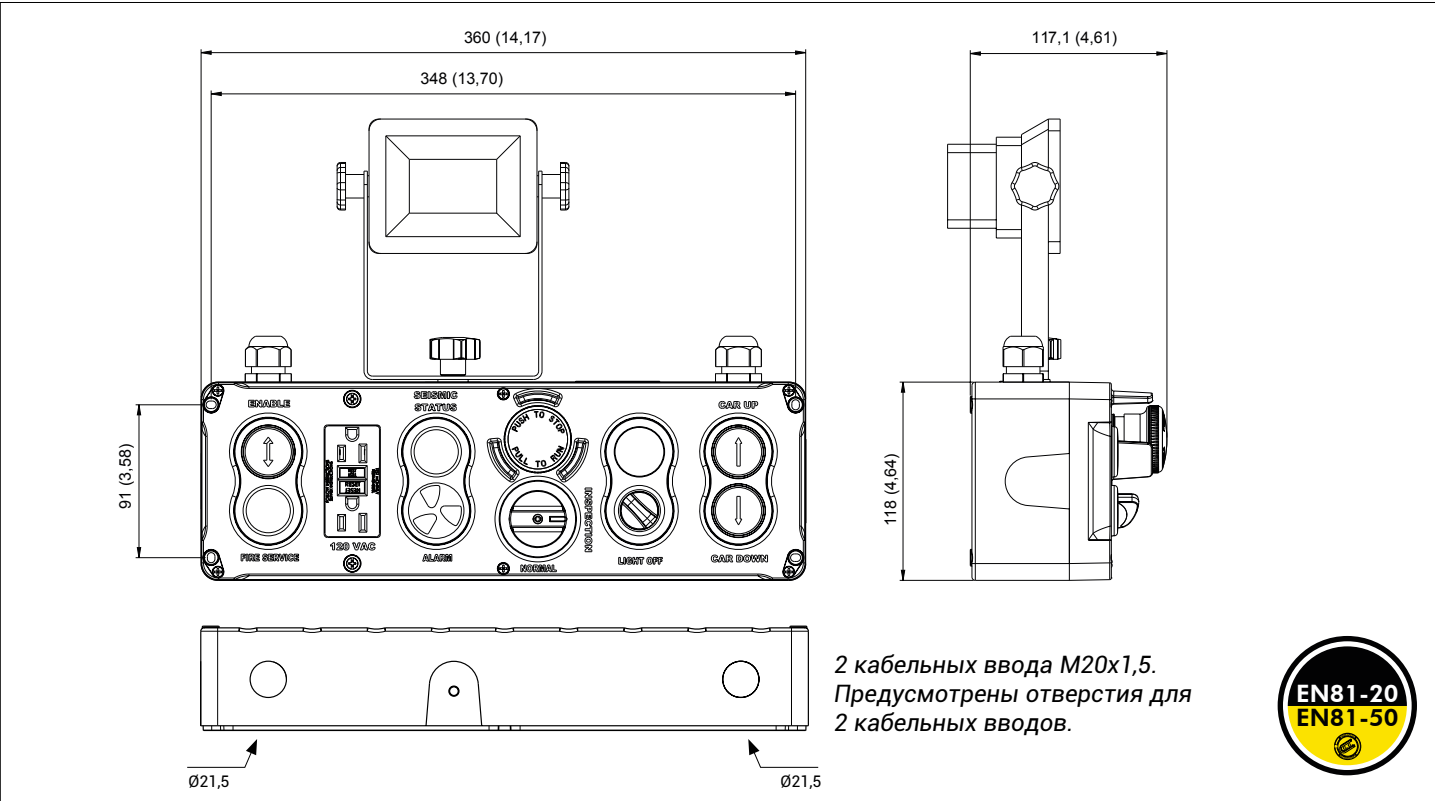
ТЕХНИЧЕСКИЙ ЧЕРТЕЖ – GMS312
