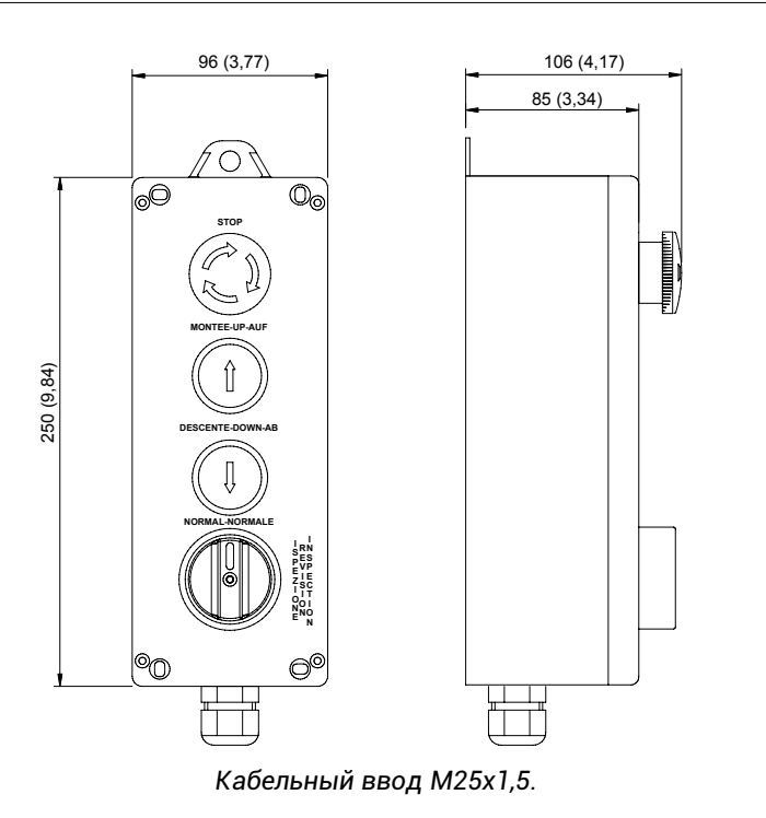
ТЕХНИЧЕСКИЙ ЧЕРТЕЖ – GM444N
