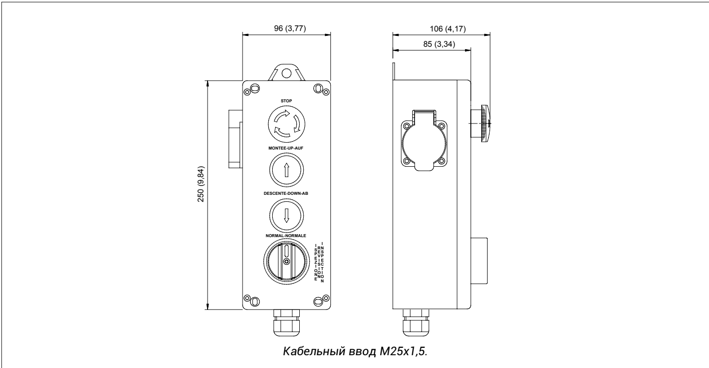
ТЕХНИЧЕСКИЙ ЧЕРТЕЖ – GM441N/..
