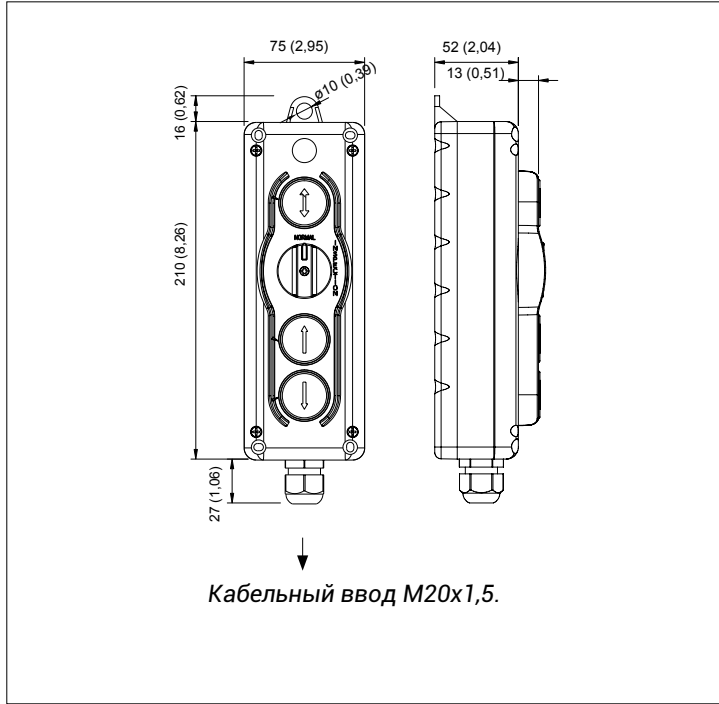
ТЕХНИЧЕСКИЙ ЧЕРТЕЖ – TLP4S006
